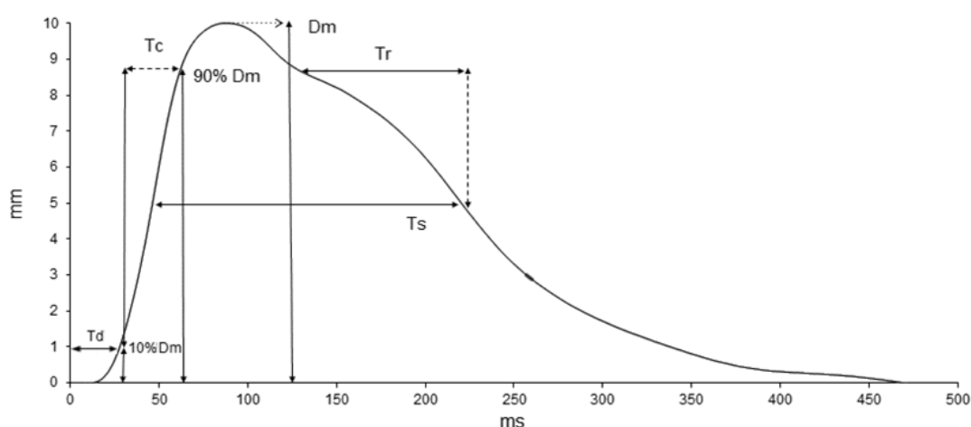
Slika 6. Shematski prikaz bočnog odgovora mišića na električni impuls sa svim pripadajućim parametrima – D_m , T_d , T_c , T_s i T_r
